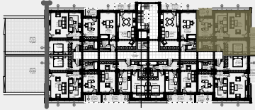
Plan etaj 2
