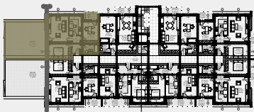
Plan etaj 2
